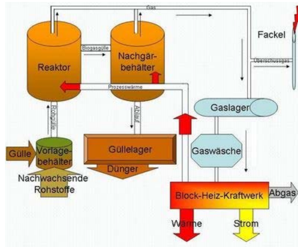
Schema einer Biogasanlage
