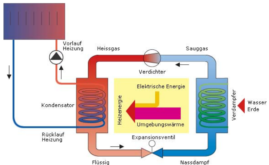
Modell Wärmepumpe
